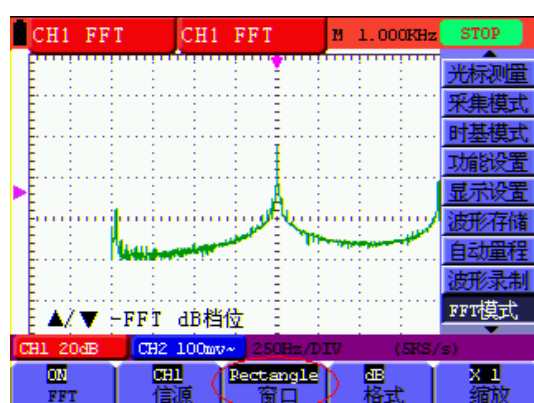
圖63. RECTANGLE 窗
