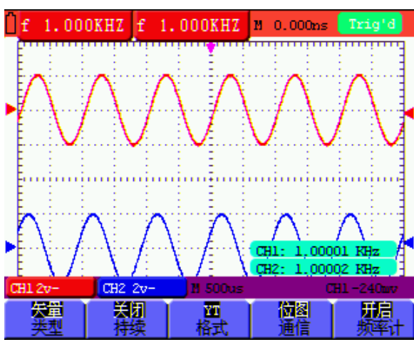
圖 48 開啟頻率計功能
