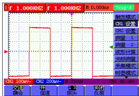
圖 17：交流耦合
