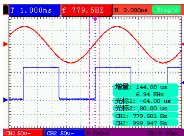
圖55：游標時間測量值
