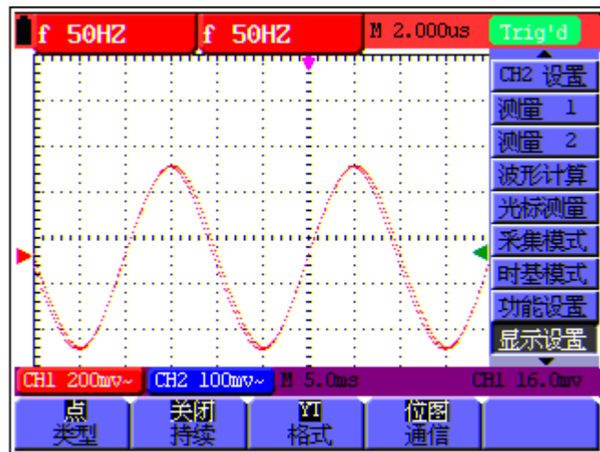
圖 46：點顯示
