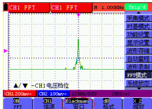
圖61. BLACKMAN窗
