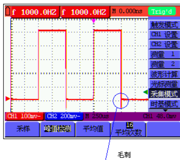
圖 16：峰值檢測
