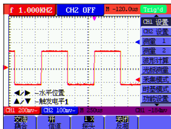
圖 35：交流耦合
