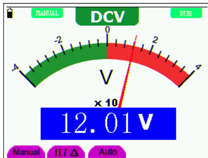
圖 33：手動/自動切換
