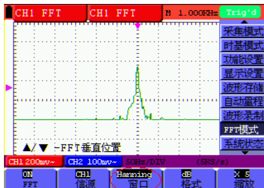
圖62. HANNING 窗
