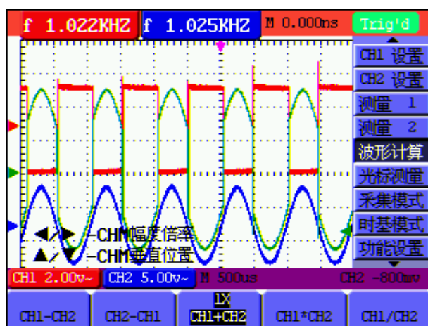
圖 19：波形計算
