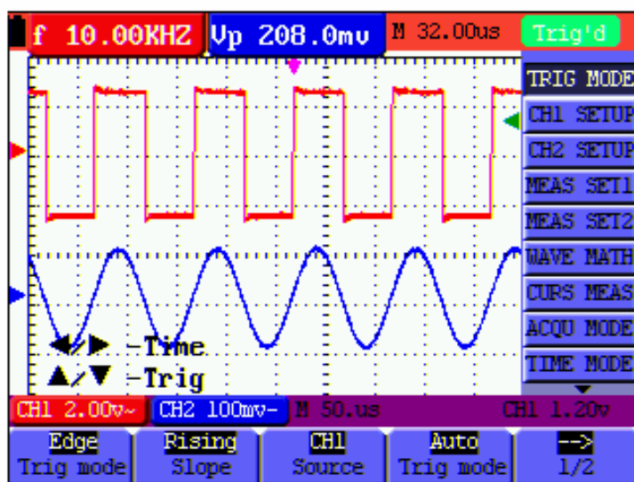
Figure 39: Edge Trigger
