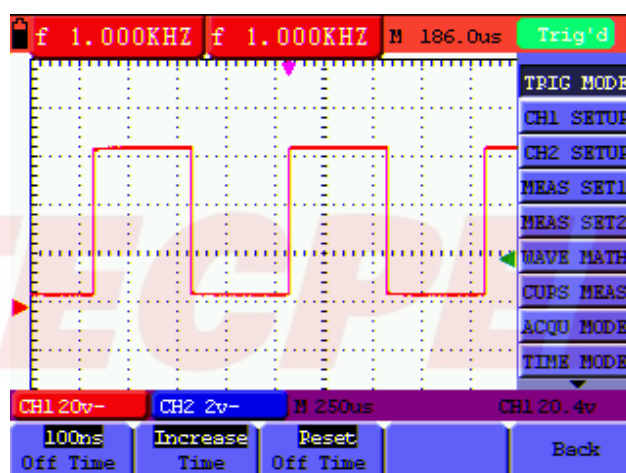
figure45:Trigger Holdoff
