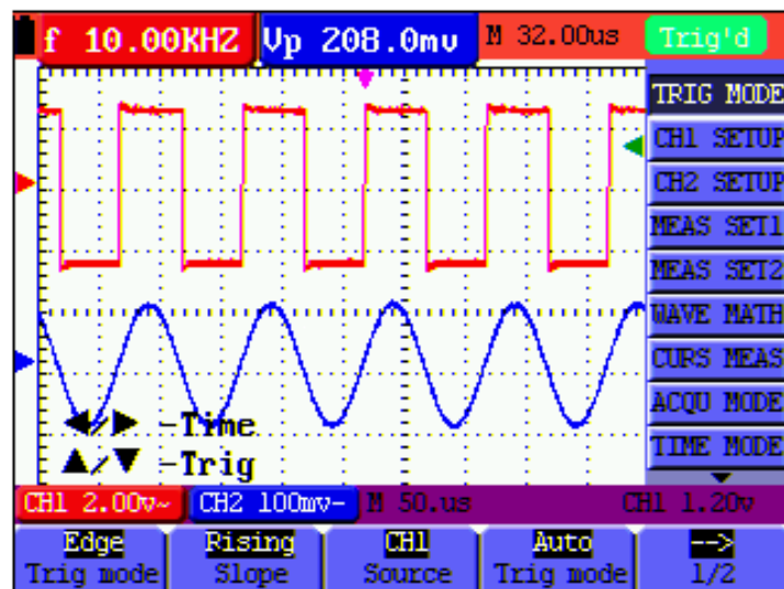
Figure 39: Edge Trigger
