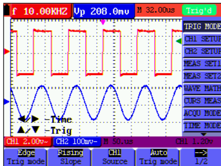
Figure 39: Edge Trigger
